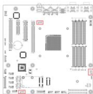
FAN: CPU 风扇/机箱风扇 1/机箱风扇 2
