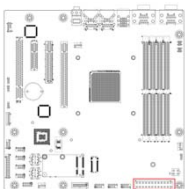
JATX1: 24Pin ATX 电源接口
