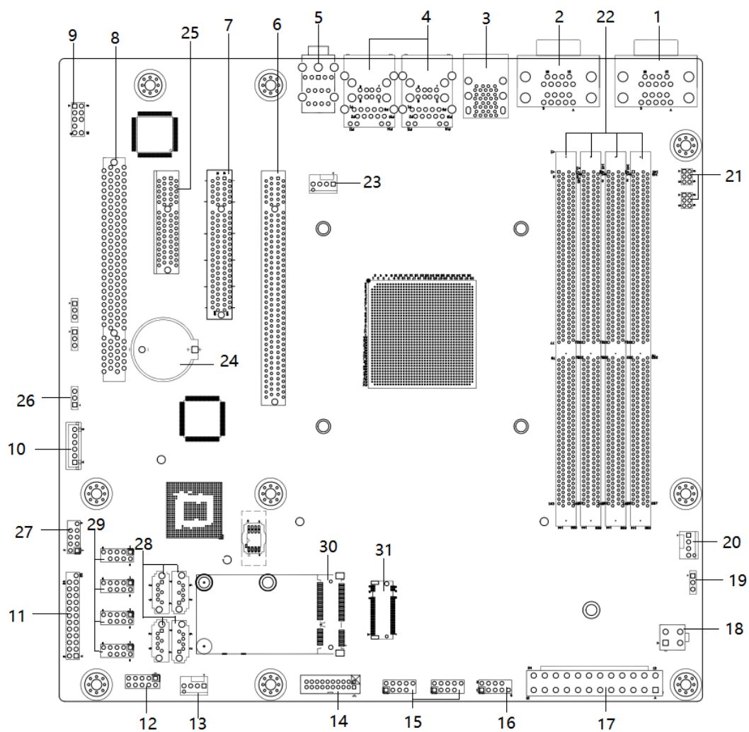
接口位置图
