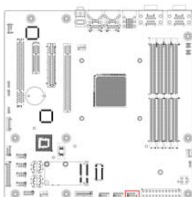
JPANEL1: 前置面板接口
